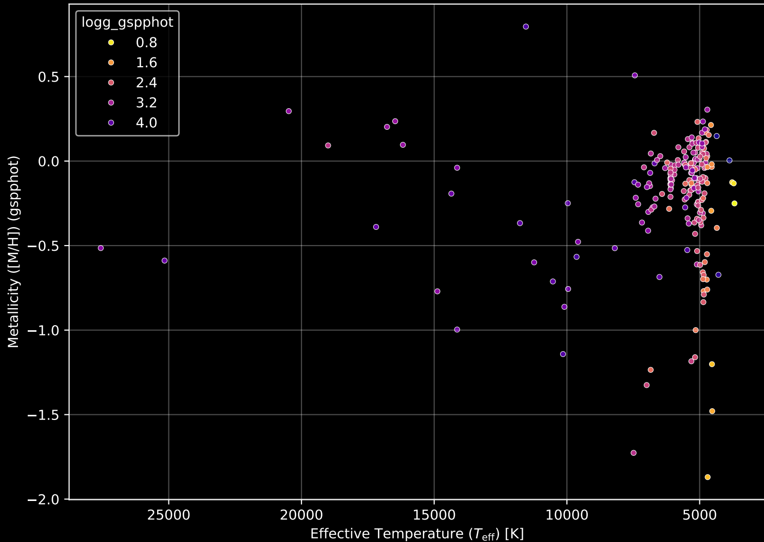
APOGEE DR17 Field: [117+01] Stellar Population Parameters (n= 210)
